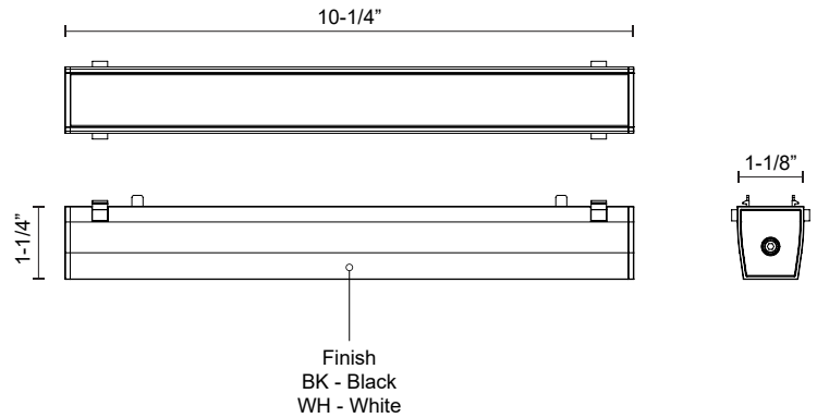
TRF17410-WH White
