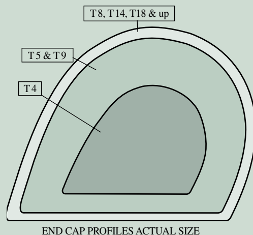
END CAP PROFILES ACTUAL SIZE
