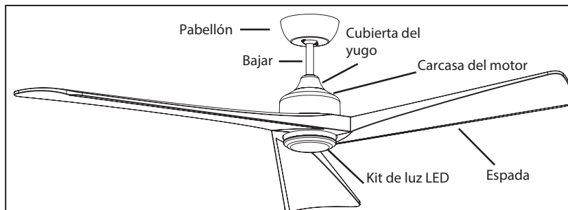
Identificación de piezas en ventilador ensamblado
