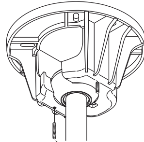
Varillas roscadas (2)
