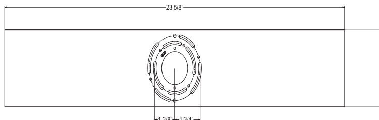
Black Plate Dimensions Fig. 3
