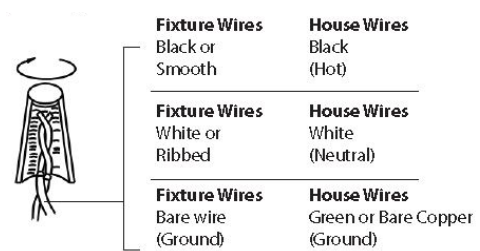
Fig. 2 Wiring
