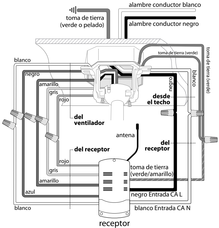
(cableado para el receptor)
