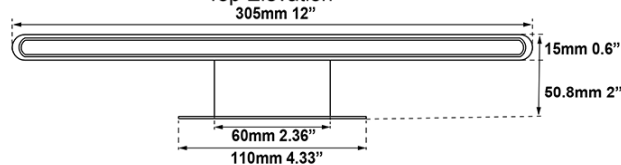
Top Elevation
