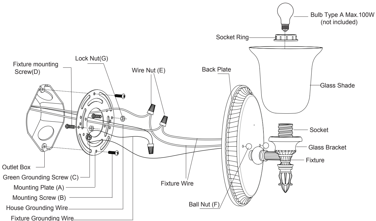
Fixture mounting Screw (D)
