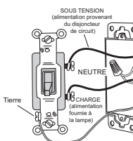
Fig. 1. Branchement typique d'un interrupteur unipolaire
