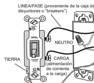
Fig. 1 Cableado Típico de un Circuito
